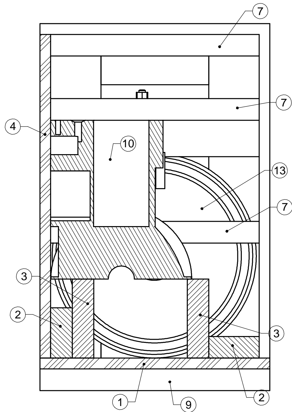
SECTION A-A
